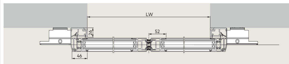
Pose sur huisserie 2 vantaux
