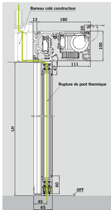
Pose sur huisserie 2 vantaux
