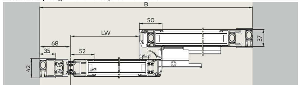
Pose dans le passage 1 vantail avec partie fixe latérale
